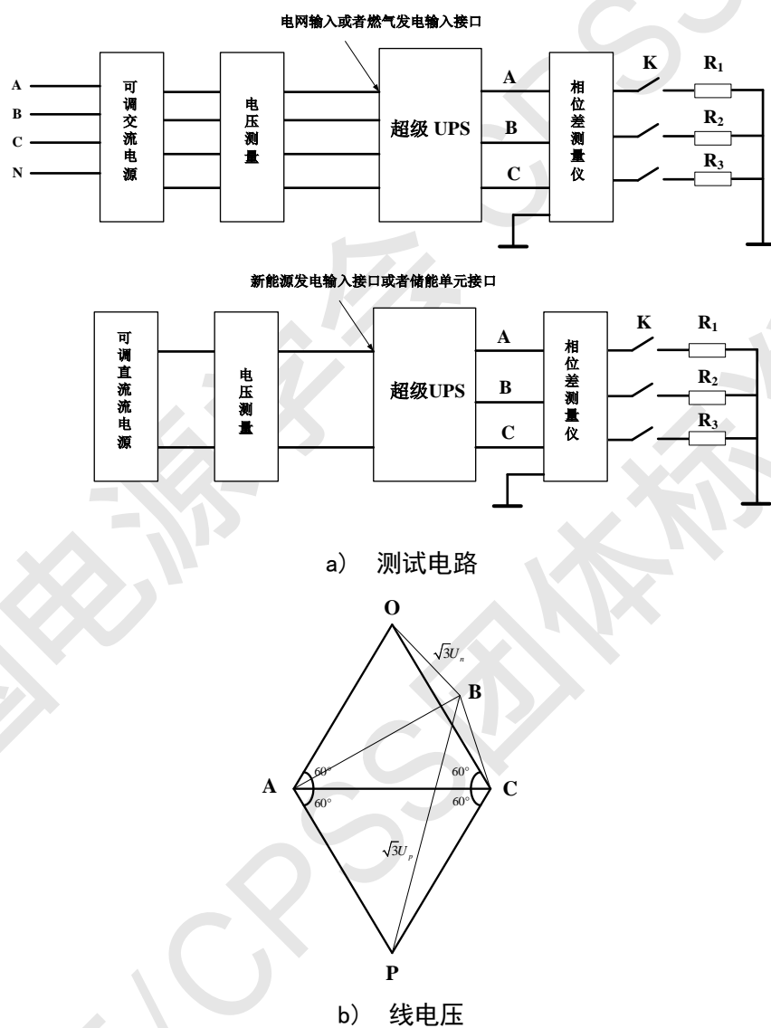
图5 电压不平衡度测试电路
