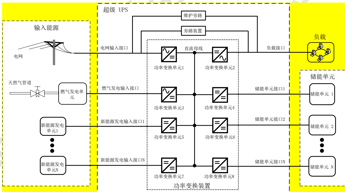
图1 超级UPS基本结构示意图
