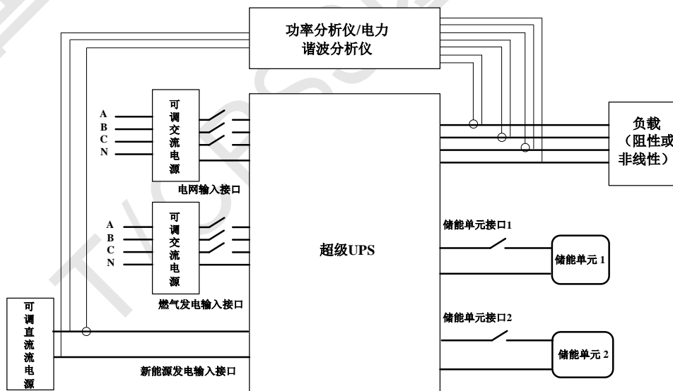
图4 新能源发电输入接口测试电路
